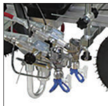
Doppia pistola per realizzare linee affiancate o di varie larghezze (TSTR8500).
